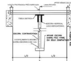
4 Det. de escoramento para vão de 10m a 12m
