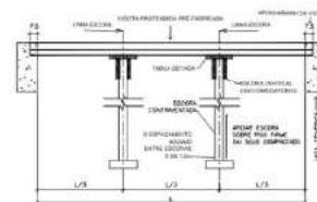
3 Det. de escoramento para vão de 6 a 10m
