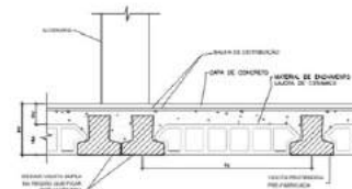
4 Det. Montagem lajes com cerâmica quando houver situação com alvenaria
